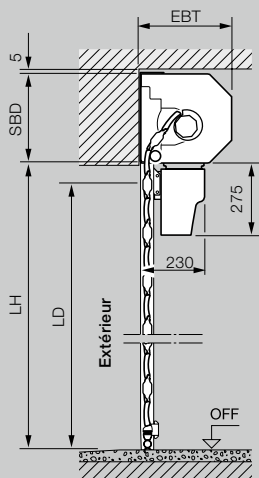
Domaine dimensionnel des portes de garage enroulables intérieures et extérieures
